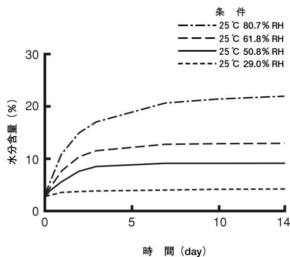
エクス粉末の吸湿曲線
