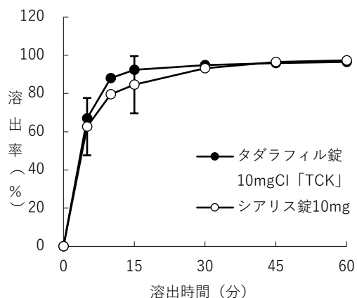
pH 4.0 (毎分 50 回転) (0.5%ポリソルベート 80 添加)
