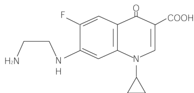
生成物〔Ⅱ〕（エチレンジアミン体）
