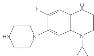
生成物〔Ⅰ〕
