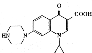
1-シクロプロピル-1,4-ジヒドロ-4-オキソ-7-(ピペラ ジンを1-イル)キノリン-3-カルボン酸 (デスフルオロ体)
