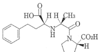
〔1〕 enalaprilate
