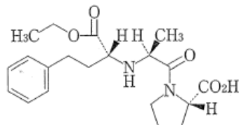
〔4〕 RSS isomer
