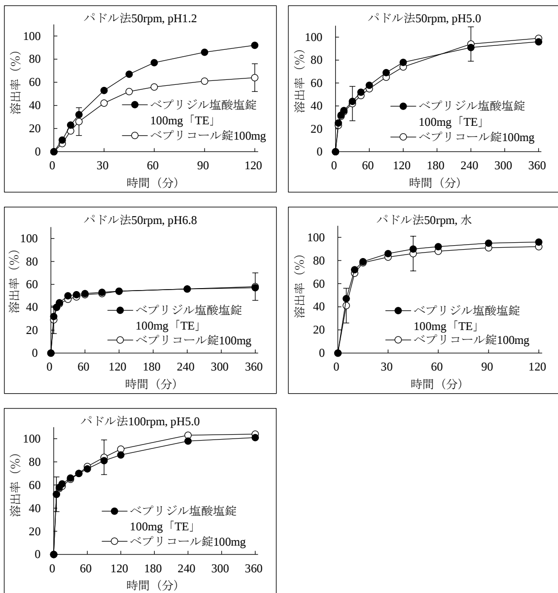
図IV-1. 各試験条件におけるベプリジル塩酸塩錠 100mg 「TE」 及びベプリコール錠 100mg の平均溶出曲線の比較 (n=12) (比較時点における標準製剤の平均溶出率 \pm 12\% 又は \pm 15\% の範囲を○で示す。)
