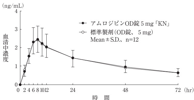
図1 5mgOD錠投与時のアムロジピンの血中濃度推移(水あり)
