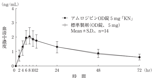
図2 5mgOD錠投与時のアムロジピンの血中濃度推移(水なし)
